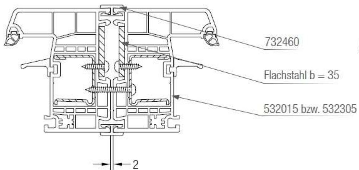
Connettore da 2 mm
